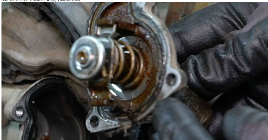
22 Pritrdišče ohišja termostata pokrijte s krpo iz mikrovlaken, da preprečite vdor umazanije in tujkov v sistem.
