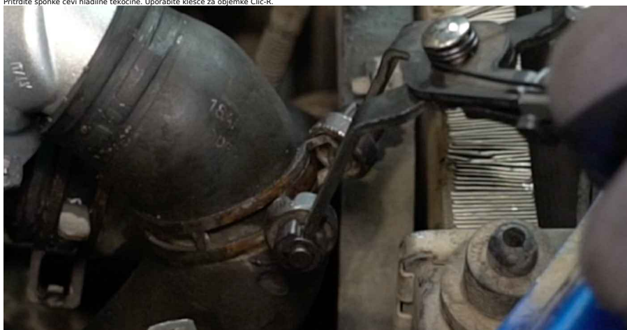
30 Očistite povezave cevi hladilne tekočine. Uporabite večnamenski čistilni sprej.
