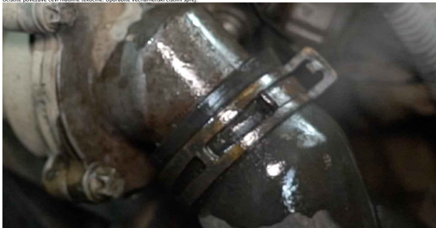
16 Sprostite sponke cevi hladilne tekočine. Uporabite kleščice za objemke Clic-R.
