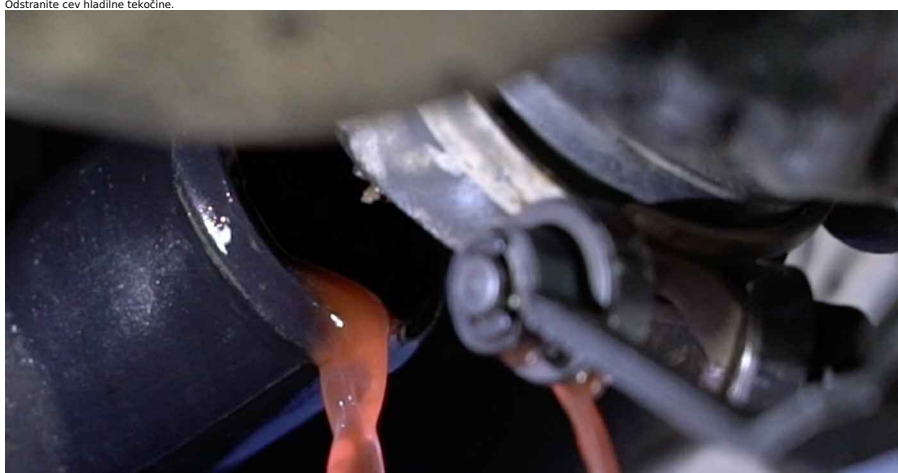
8 Odstranite cev hladilne tekočine.
