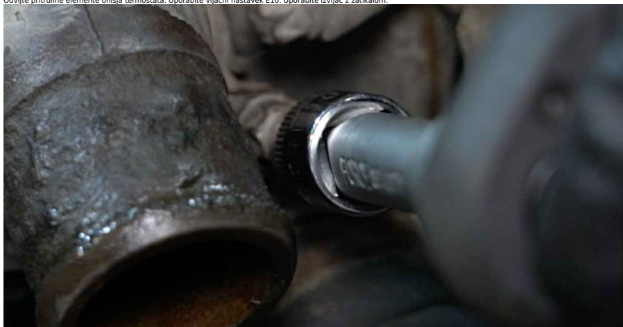
21 Odstranite ohišje termostata skupaj s termostatom.
